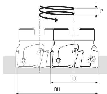
interpolacja śrubowa / helical interpolation
