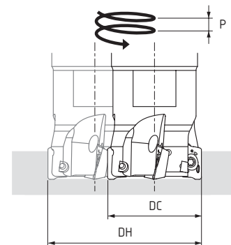
interpolacja śrubowa / helical interpolation
