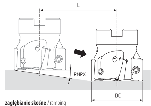
zagłębianie skośne / ramping
