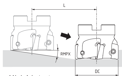
zagłębianie skośne / ramping
