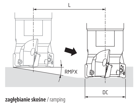
zagłębianie skośne / ramping
